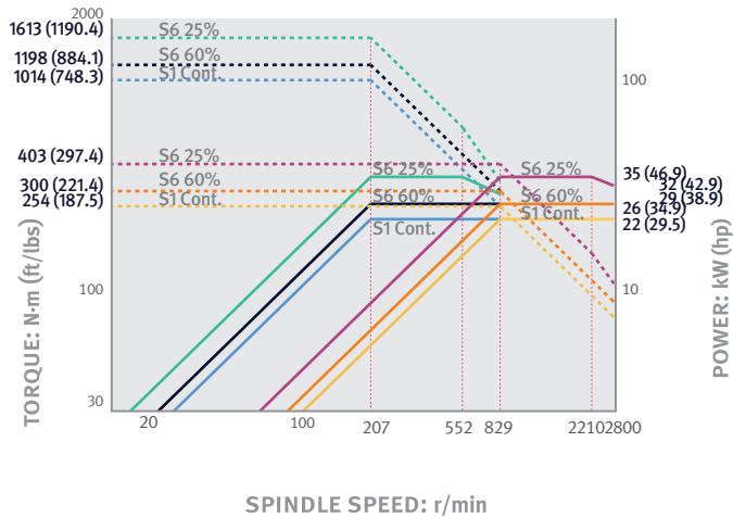
PUMA GT3100, PUMA GT3100L / DOOSAN FANUC i
