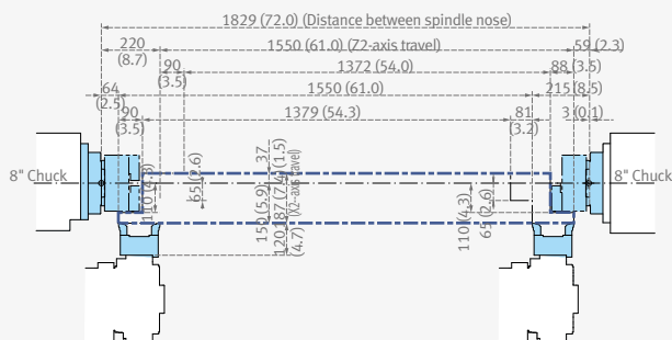
Double OD Tool holder
